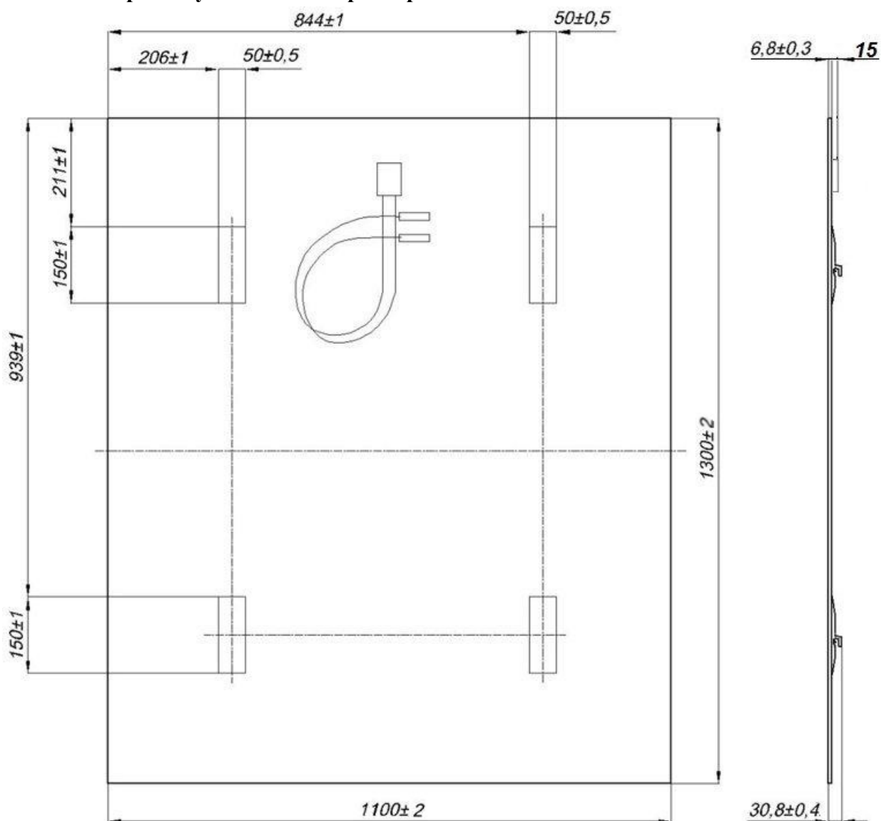
Рисунок 1 Габаритно-установочные размеры ФЭМ
