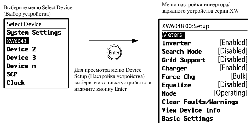
Рис. 2-4 Выбор меню Device Setup (Настройка устройства)
