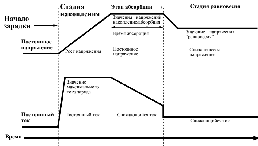
Рис. 3-4 Трехступенчатый цикл зарядки аккумуляторов
