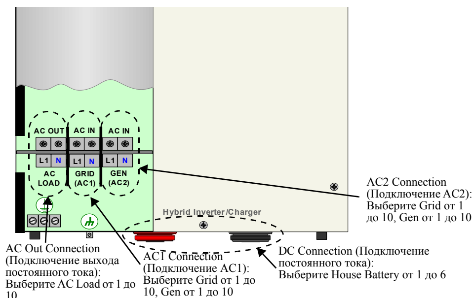
Рис. 3-8 Представление подключений инвертора/зарядного устройства серии XW
