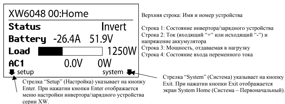
Рис. 2-6 Первоначальный экран инвертора/зарядного устройства серии XW
