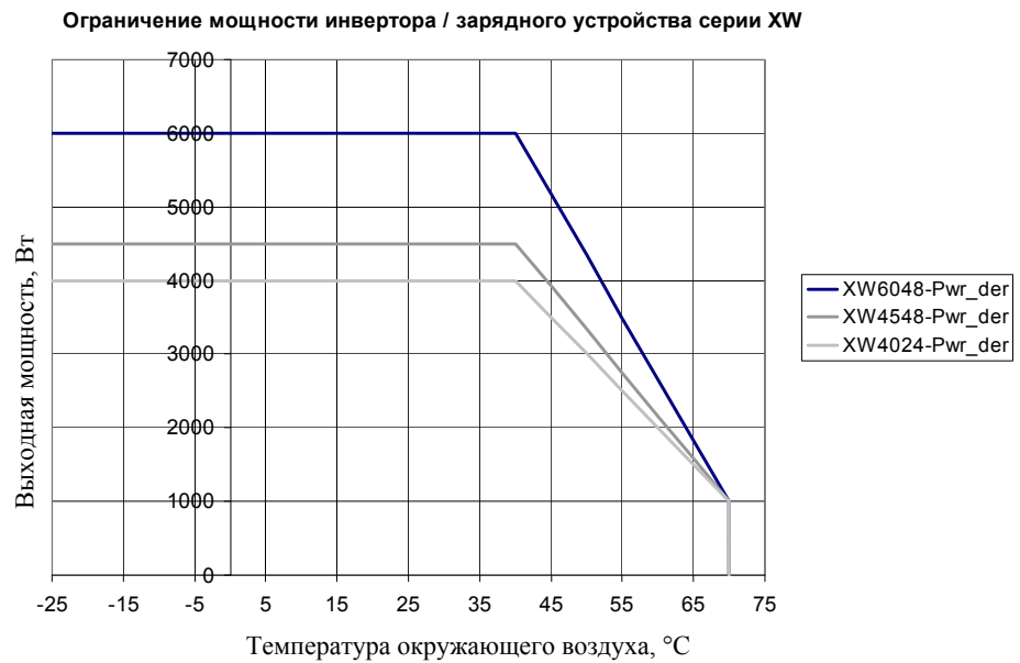
Рис. А-2 Зависимость выходной мощности от окружающей температуры
