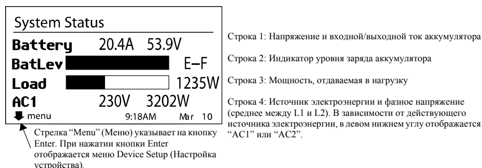
Рис. 2-5 Экран System Status (Состояние системы)
