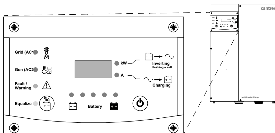
Рис. 1-1 Информационная панель инвертора
